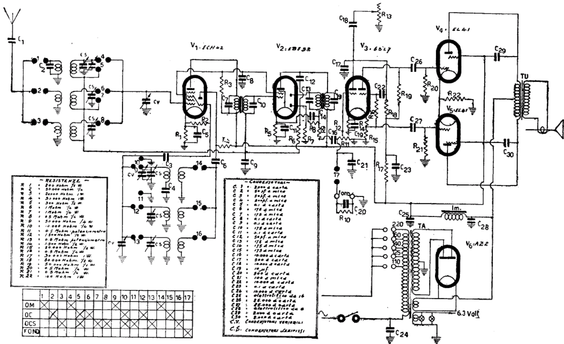
INCAR - Mod. VZ 601 - Medie e due corte. EBF32 amplif. MF e rivelatrice. 6SL7 amplificatrice di tensione con un triodo, e invertitrice di fase a catodo seguitatore con l'altro triodo. Resa d'uscita 9 watt.
